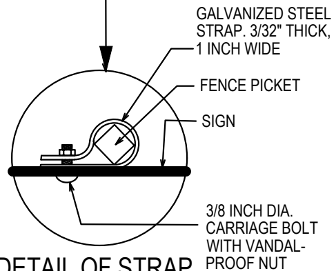
DETAIL OF STRAP N.T.S.
